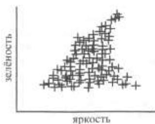
Рис. 1. Графическое представление преобразования «шапочка с кисточкой».
