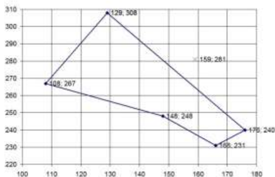
Рисунок 4 – Графы минимальных расстояний.
